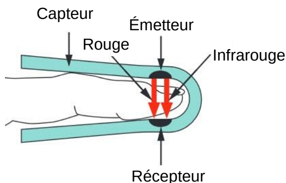
Figure 4 : schéma du capteur
