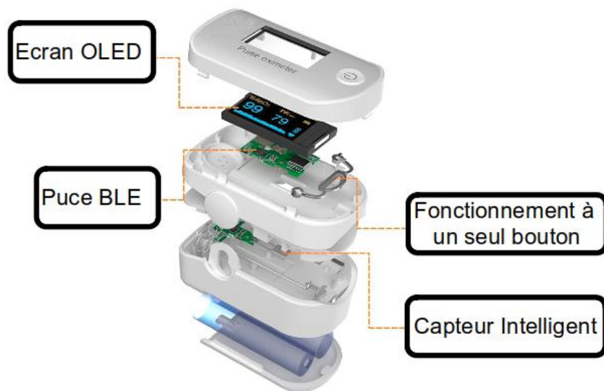
Figure 1 : vue éclatée d'un oxymètre de pouls
