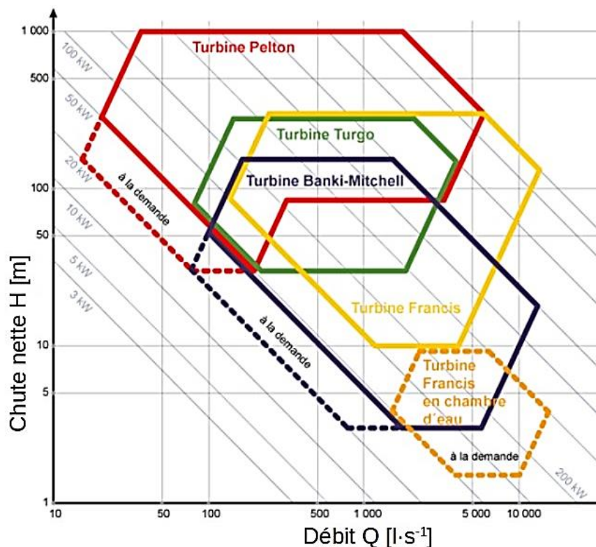
Figure 2 : schéma de sélection d'une turbine en fonction de la hauteur et du débit de la chute (source université de Perpignan CC-BY-NC-SA)
