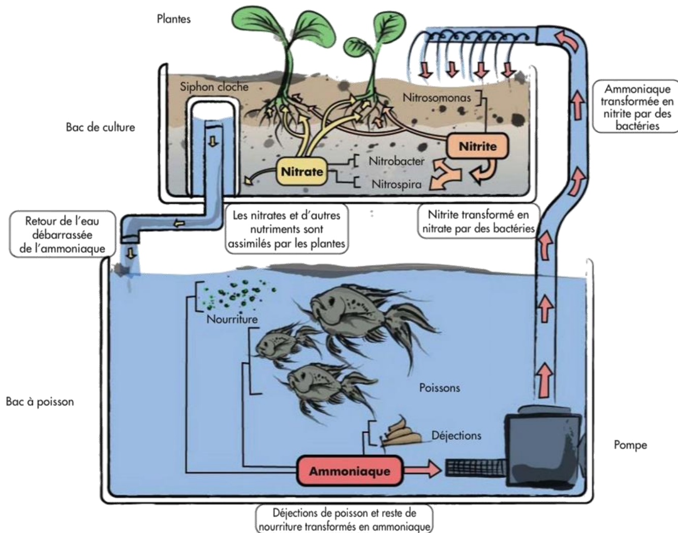
Figure 2 : principe de fonctionnement d'une installation aquaponique
