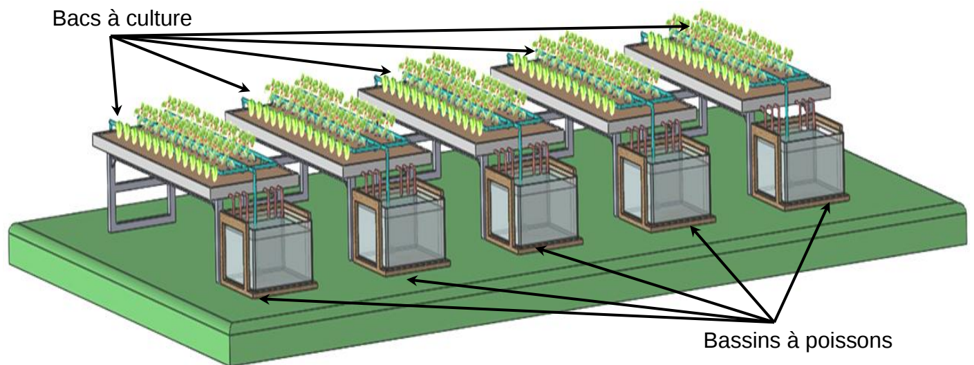
Figure 1 : ferme aquaponique après agrandissement
