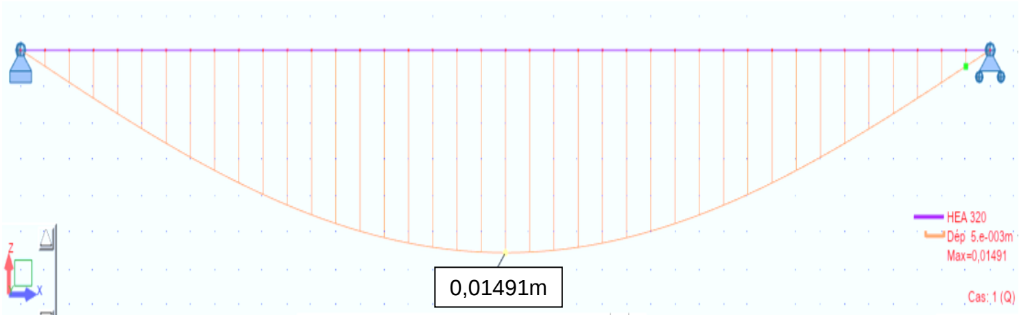
Figure 5 : simulation numérique de la flèche
