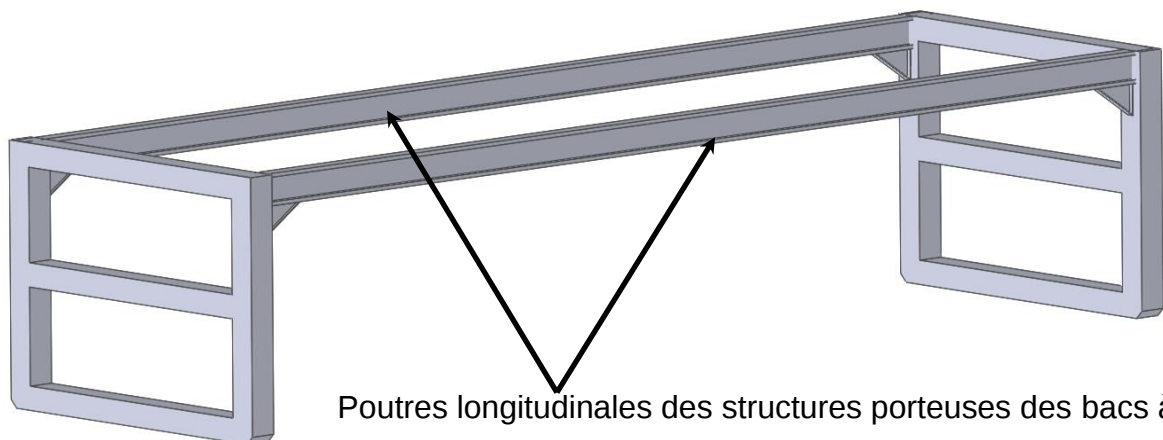
Figure 4 : structure porteuse des bacs à culture
