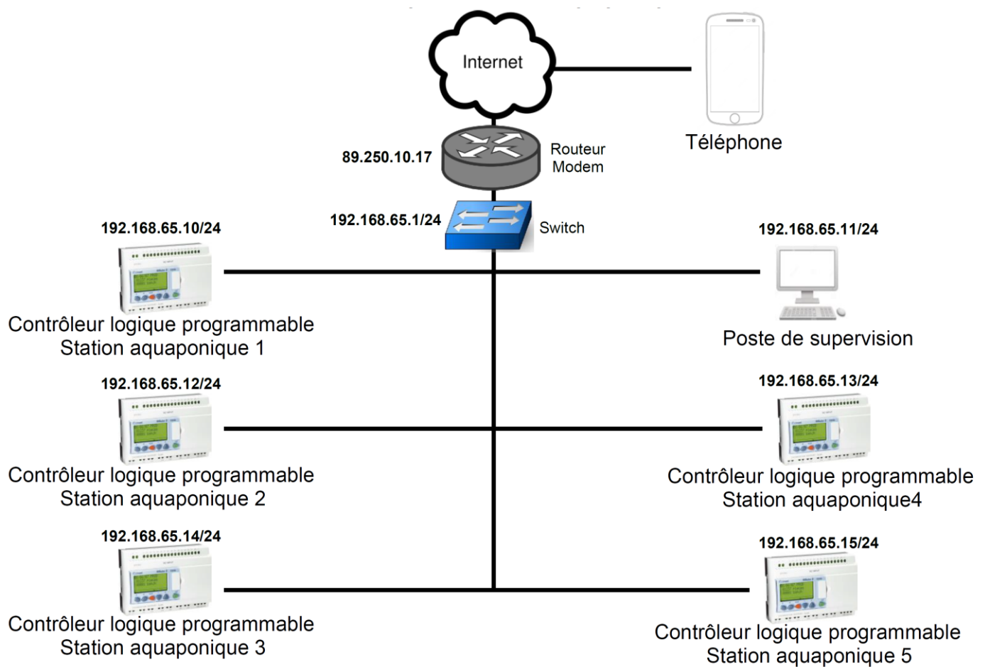
Figure 8 : structure du réseau informatique de la ferme aquaponique
