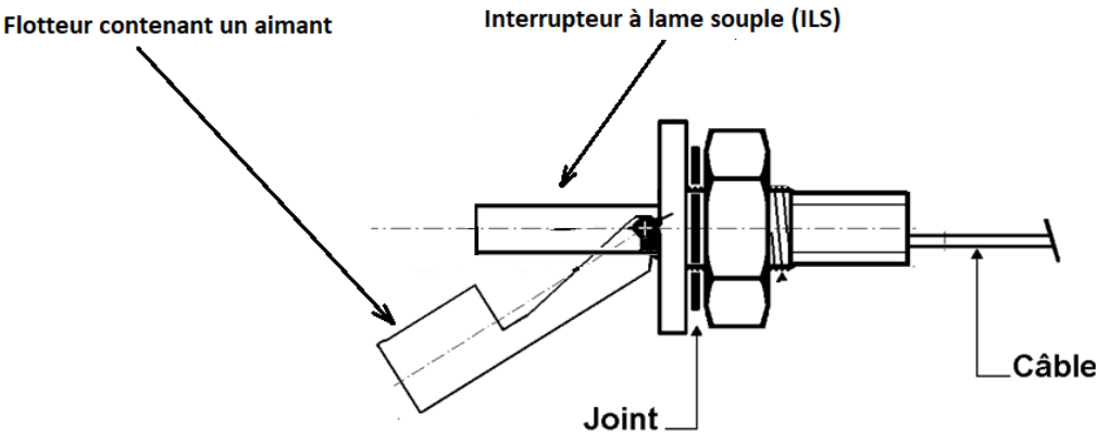
Figure 6 : fonctionnement des capteurs à flotteur
