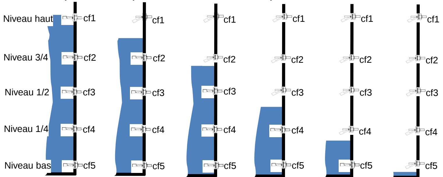
Figure 7 : détection du niveau d'eau dans les bacs à poissons
