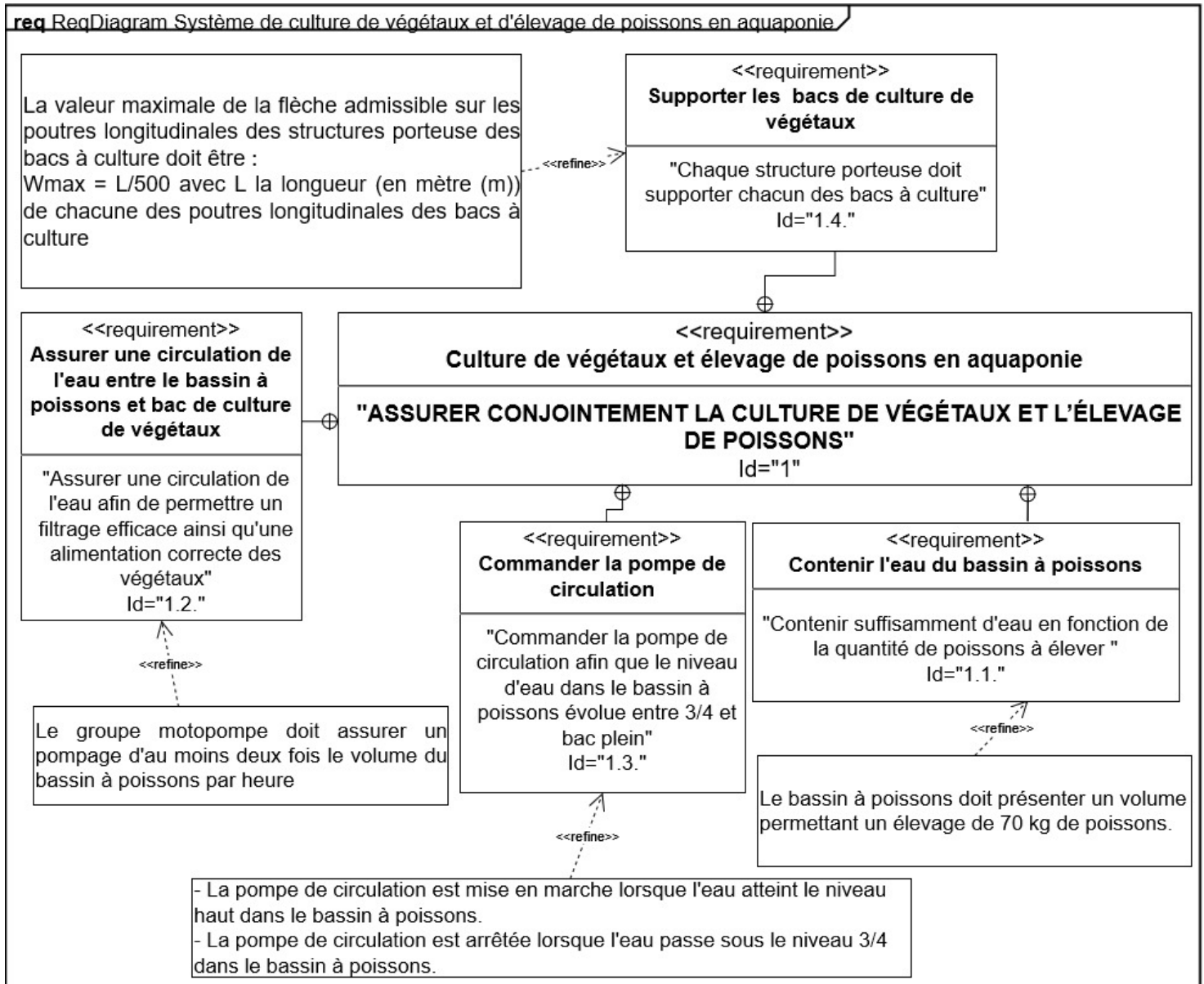
Figure 3 : diagramme des exigences de la ferme aquaponique
