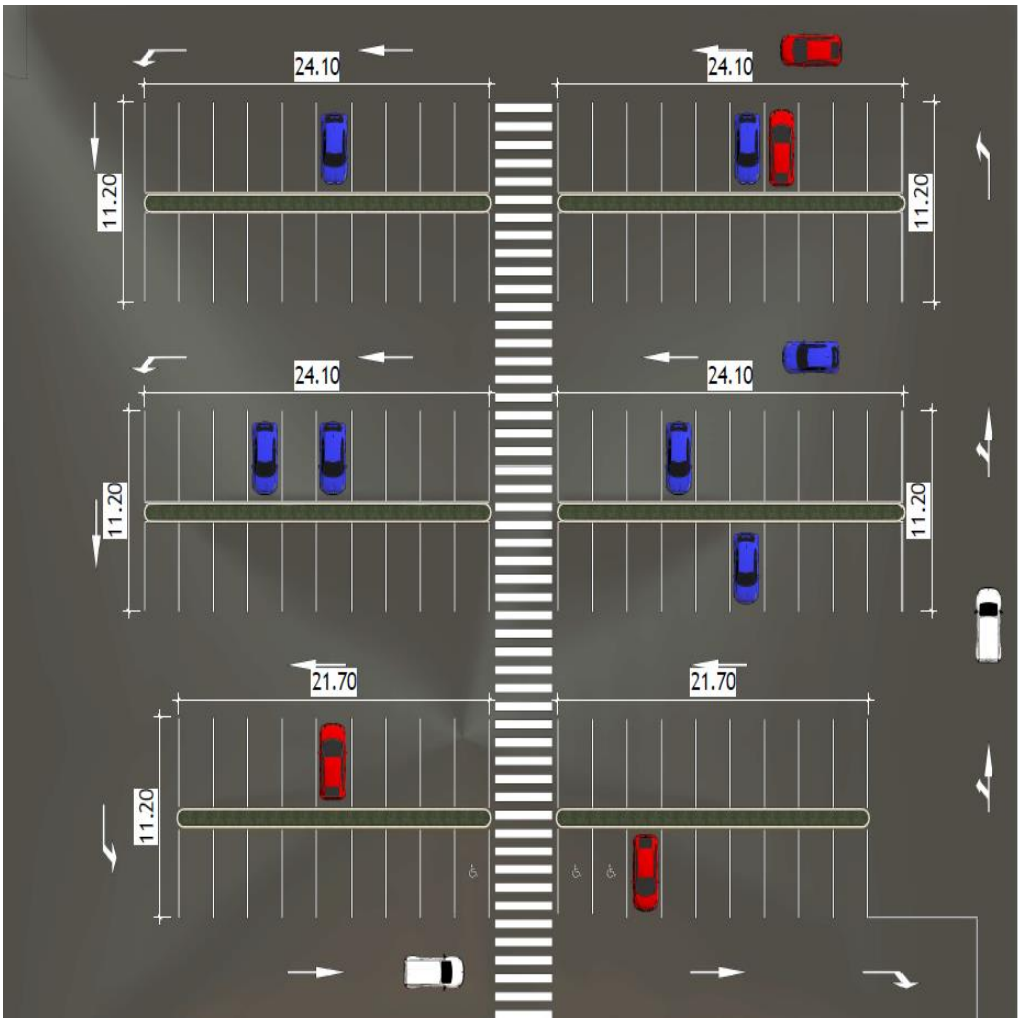
Figure 5 : plan de masse du parking
