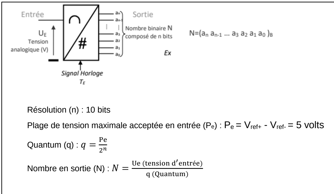
Fig. 4 – Caractéristiques du convertisseur analogique/numérique (CAN)
