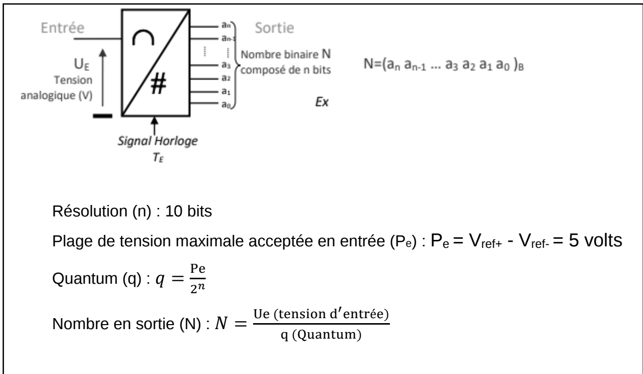
Fig. 4 – Caractéristiques du convertisseur analogique/numérique (CAN)
