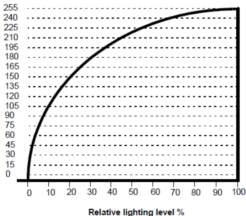
Caractéristiques de gradation du bus DALI
