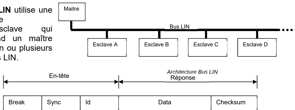
Trame de message LIN
