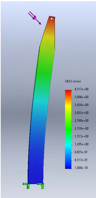
Déplacements (flèche)
