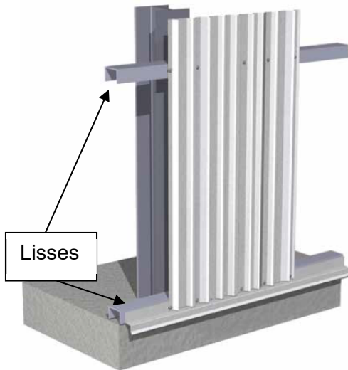
Bardage vertical simple peau
