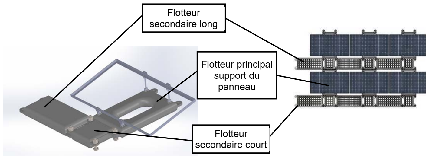
Figure 3 : Système flottant, principe d'un module et vue de dessus d'une série de 6 modules accolés sur site
