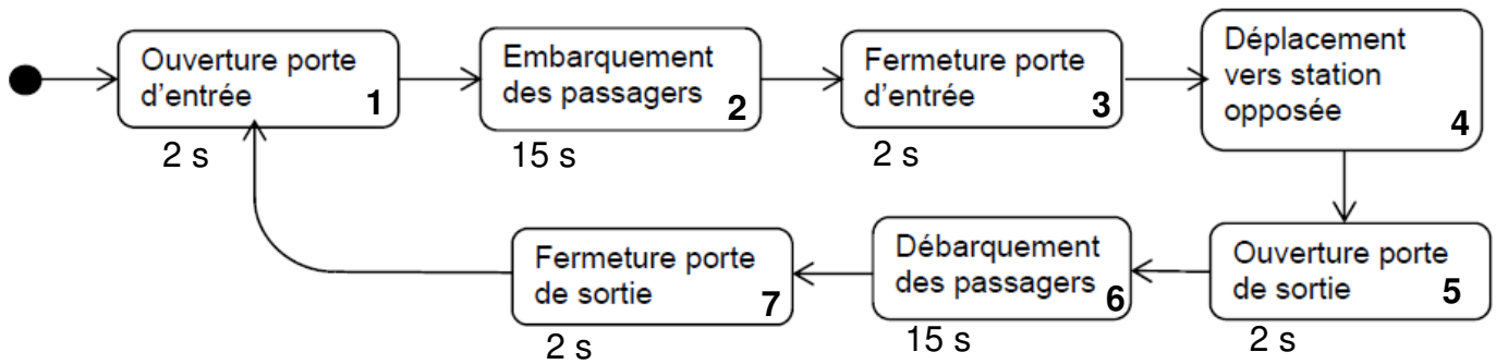
Figure 3 : diagramme d'état du cycle de fonctionnement
