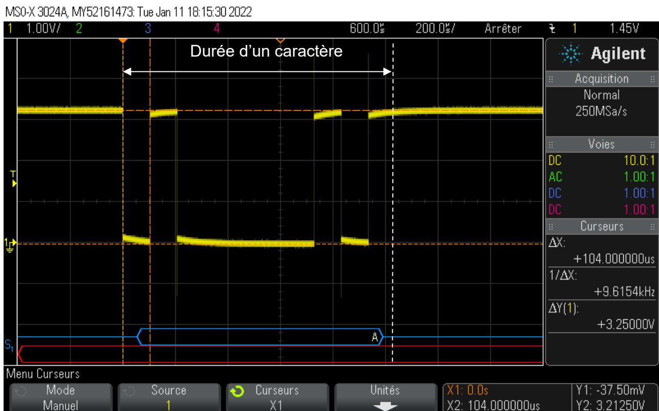
Figure 3 : signaux échangés entre le PIC18F4423 et le module XBee.
