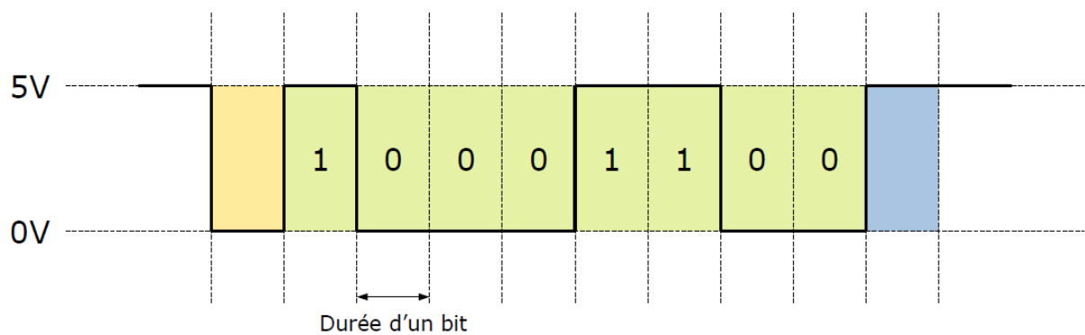
Figure 4 : exemple de trame sur notre liaison série.
