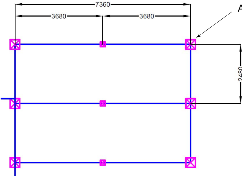
Détail des bungalows de type C pour dessin de la surface d'influence
