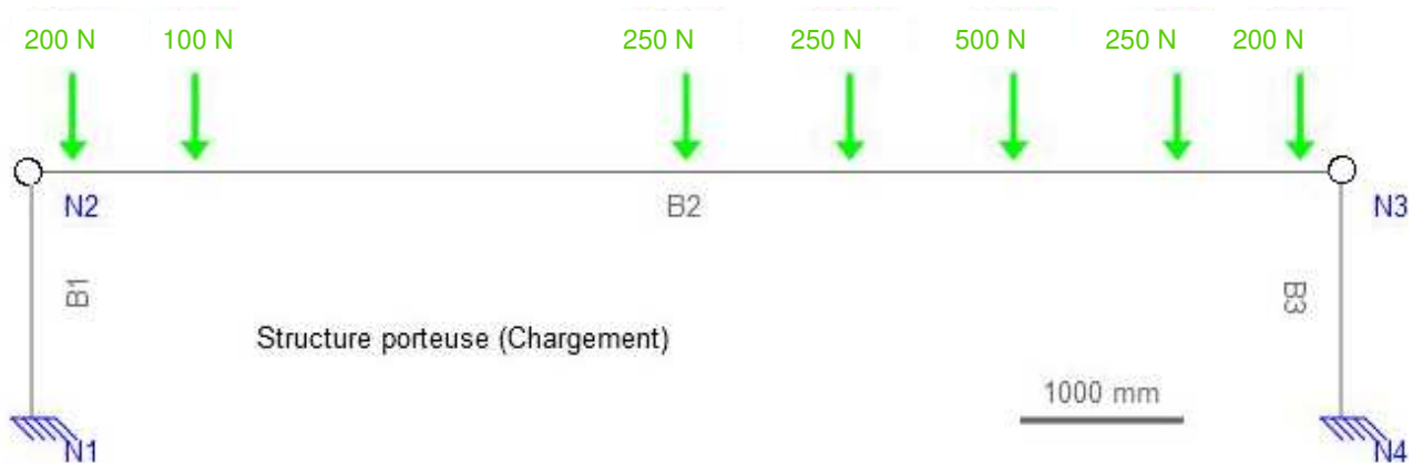
Figure 1 : modélisation de la structure porteuse
