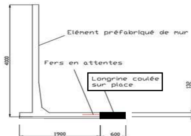
Modélisation mur de soutènement (vue en coupe)
