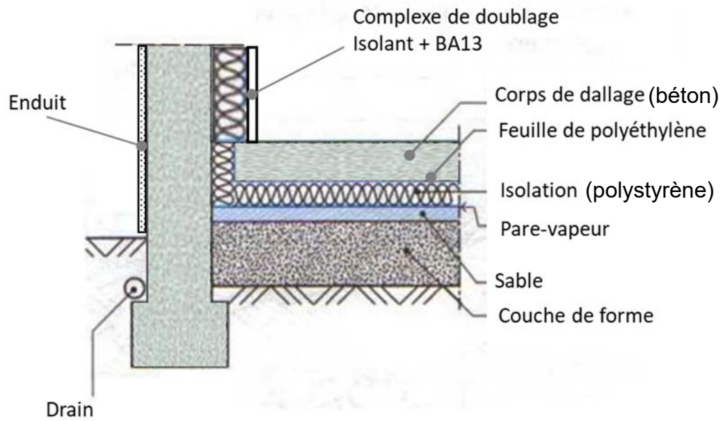
DTS1b : coupe de principe sur les fondations
