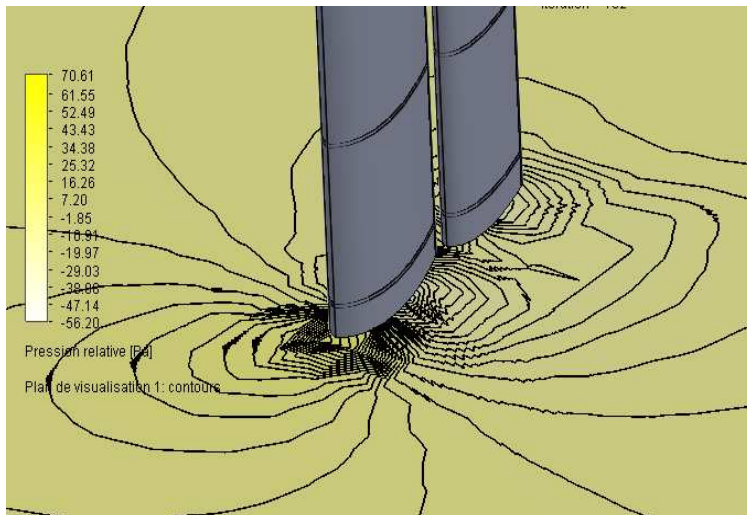
Simulation de l'écoulement du fluide autour du propulseur éolien.
