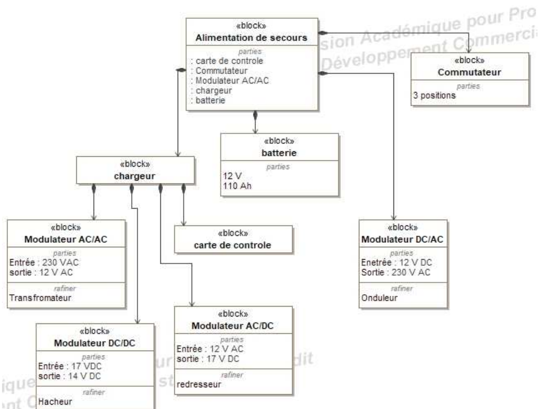
Diagramme B.D.D.
