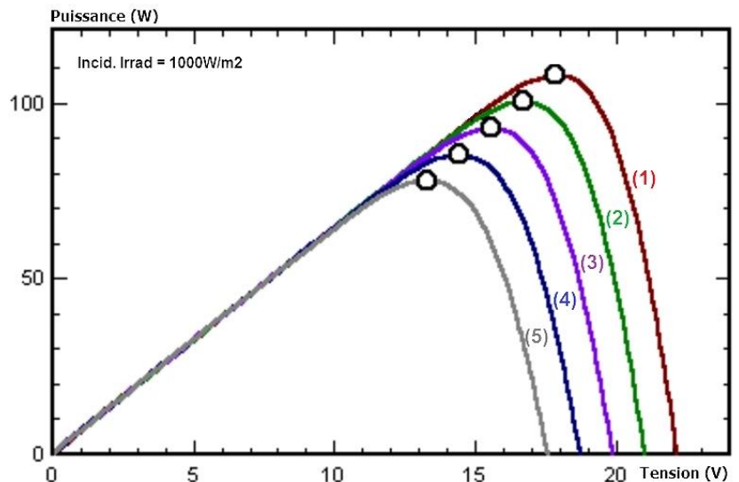
Courbe Pcrête en fonction de la température pour un panneau de 100W.
