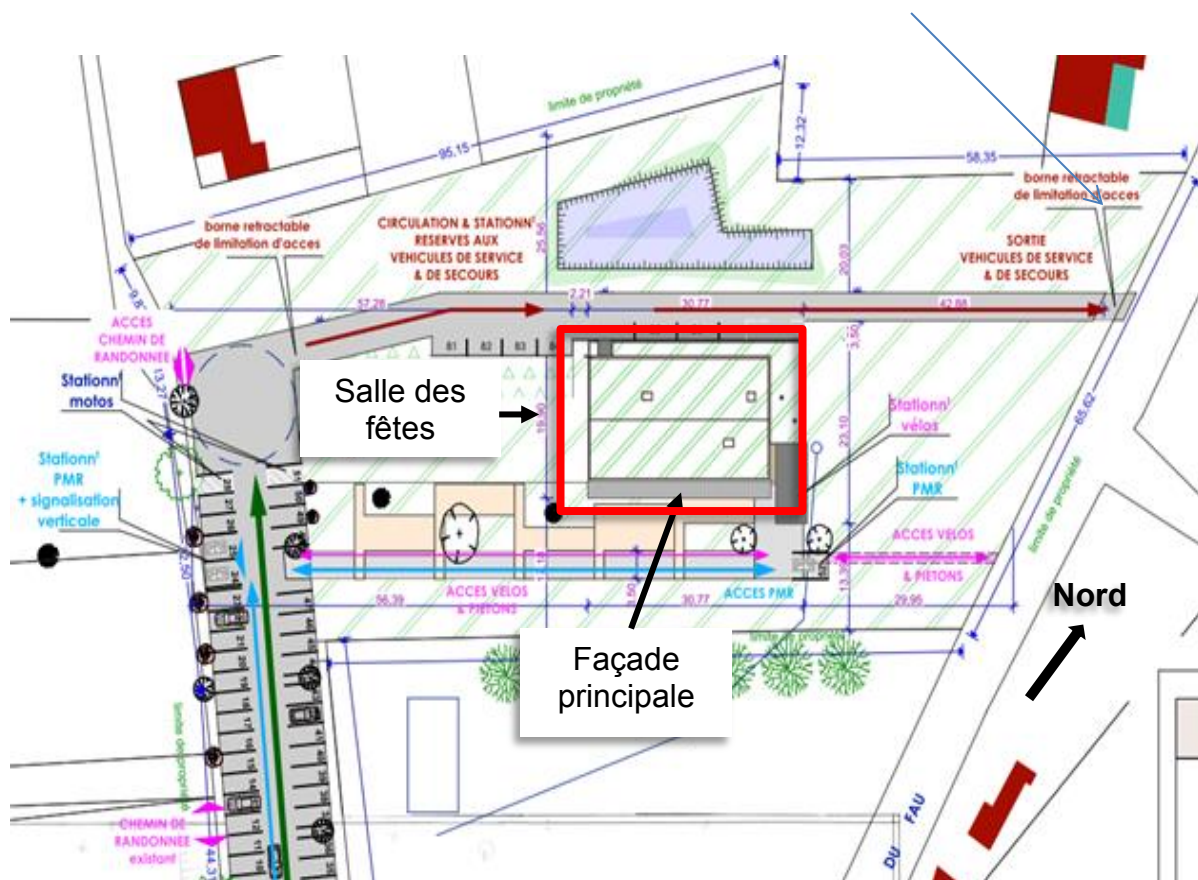
Figure 3 : plan de masse de la salle des fêtes
