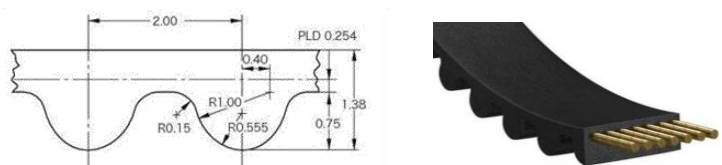
Figure 14 : Caractéristiques courroie synchrone GT2
