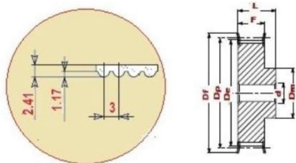
Figure 8 : Poulie crantée
