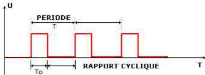
Figure 9 : Chronogramme d'un signal PWM
