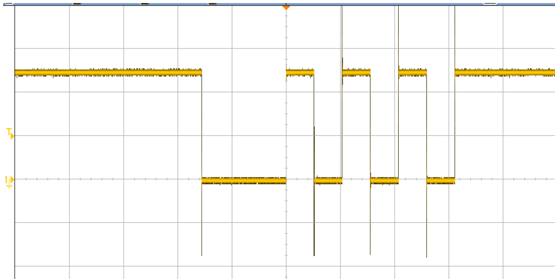
Figure 5 : Trame de commande envoyée au slider
