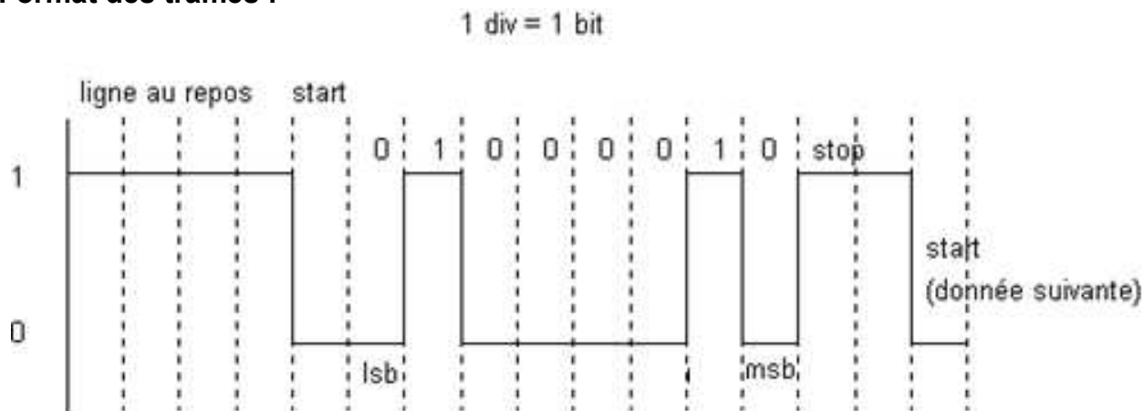
Figure 10 : Format d'une trame
